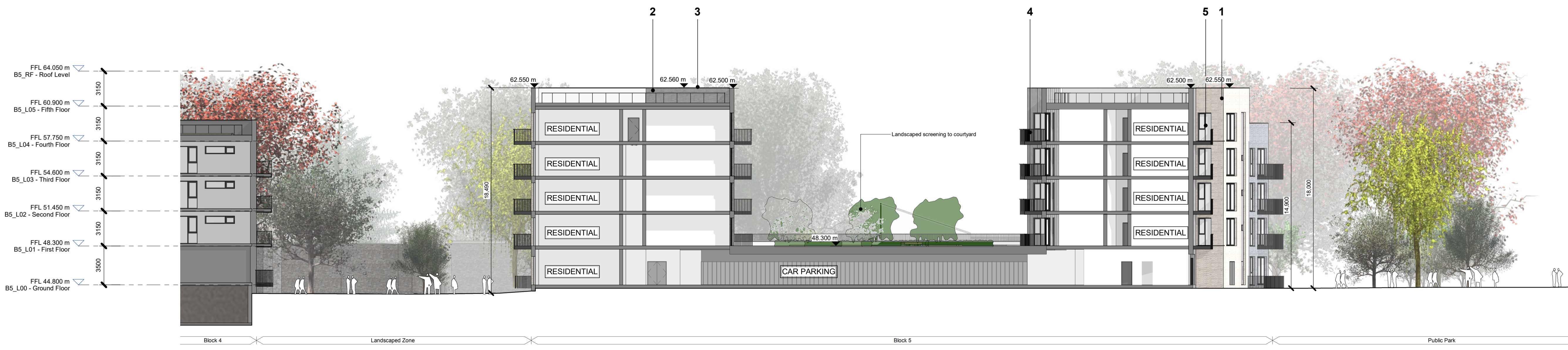
Block 05, E/W Section 02 1 : 200
